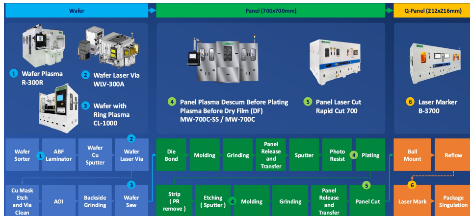
鈦昇之面板級封裝解決方案
